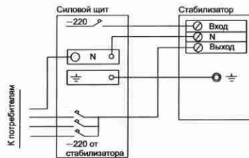
Рисунок 1 – Схема электрических соединений
