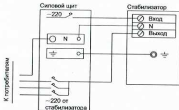
Рисунок 1 – Схема электрических соединений
